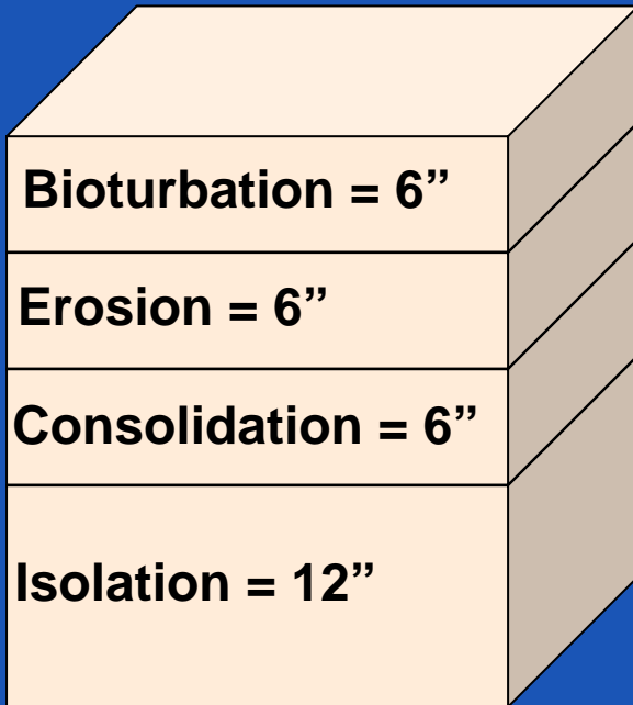
Sand Cap
